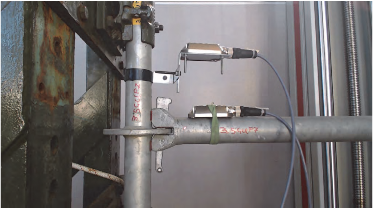
Figura 3-155 Foto inizio prova
