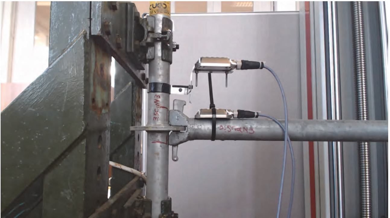
Figura 3-119 Foto inizio prova
