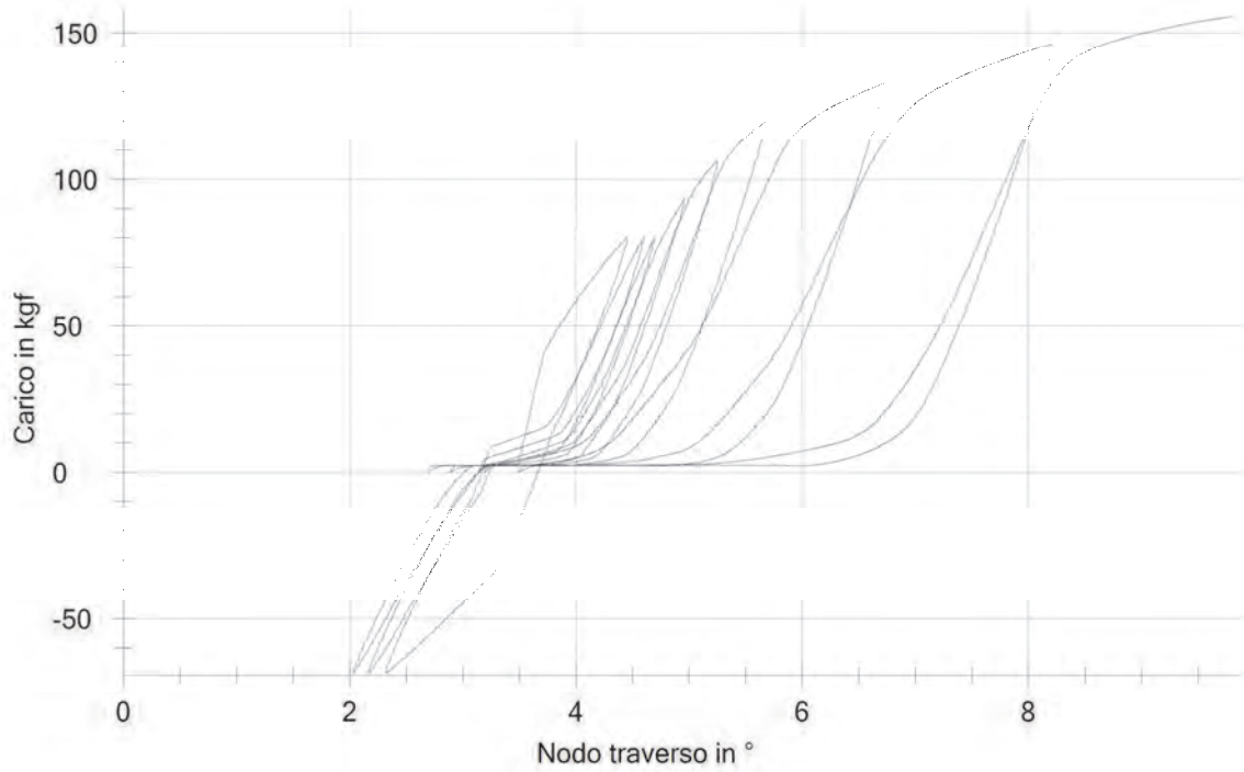
Figura 3-135 Curva carico – inclinazione trasverso al nodo
