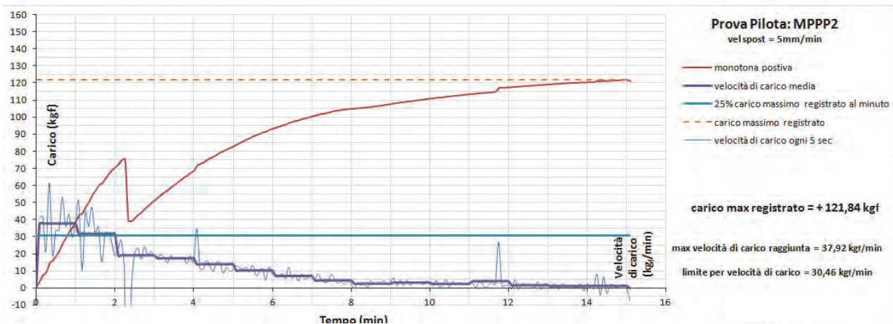
Figura 3-24 Curva carico-tempo. Velocità di carico media (kg/min). Limite per la velocità di carico calcolato in base al massimo carico registrato
