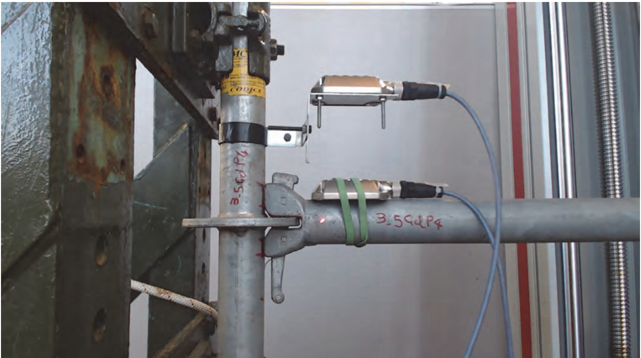
Figura 3-143 Foto inizio prova
