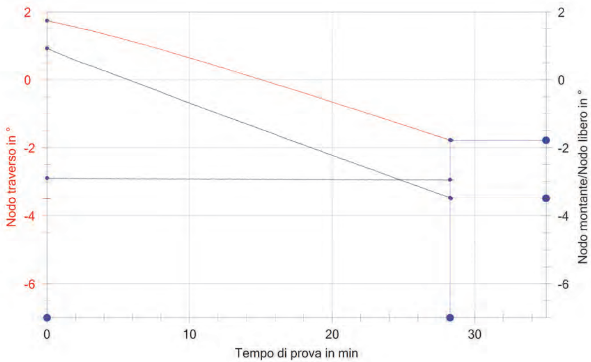
Figura 3-40 Inclinazione nodo trasverso, nodo libero e nodo montante nel tempo
