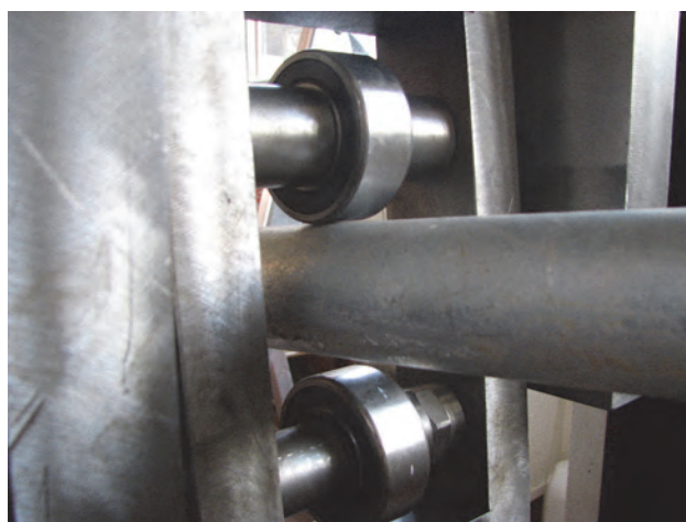
Figura 3-3 Accessorio per il trasferimento dello spostamento della traversa della macchina di prova al traverso del dispositivo di collegamento sottoposto a prova
