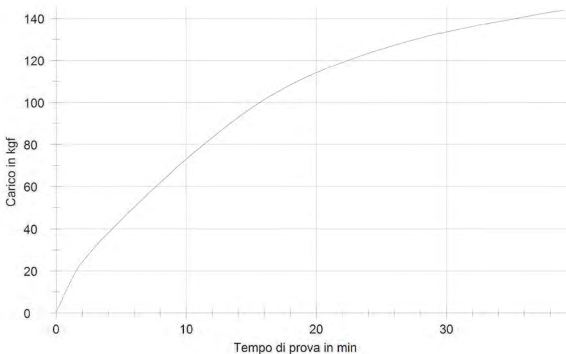
Figura 3-91 Curva carico-tempo.
