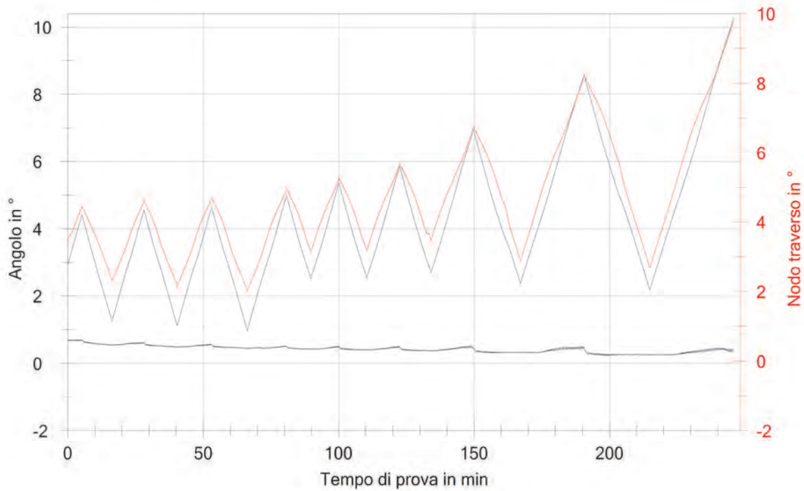
Figura 3-136 Inclinazione nodo trasverso, nodo libero e nodo montante nel tempo
