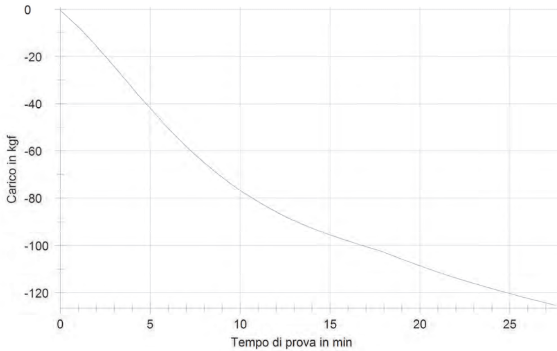
Figura 3-49 Curva carico-tempo.
