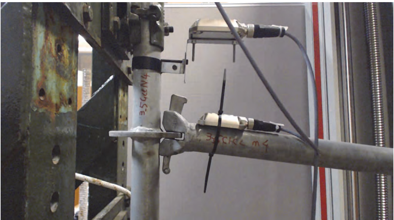
Figura 3-126 Foto fine prova
